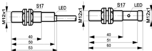
wyjście kablowe
