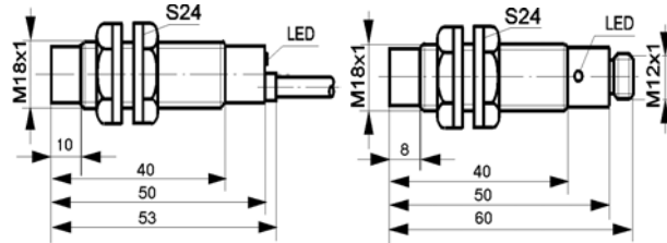
wyjście kablowe
