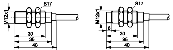
Czoło wbudowane
