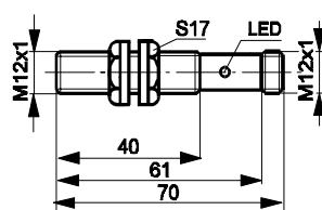
wyjście konektorowe
