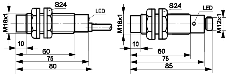
wyjscie kablowe
